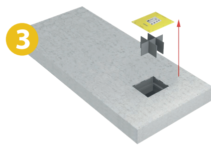
3 Décoffrage du couvercle et des renforts de la RÉZABOITE CV
